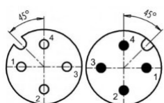
Mastkabel für Gabelstapler M12-A-5p +6x offene Litzen Mast cable for Forklift M12-A-5p + 6x open wire
