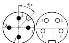
Adapter M12-A-M-5p auf M16-F-4p Adapter M12-A-M-5p auf M16-F-4p
