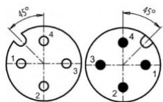
Verbindungskabel M12A/4p Connection cable M12A/4p
