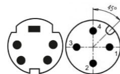
Verbindungskabel MiniDIN-M-4p auf M12-A-M-5p (MK320) Connection cable MiniDIN-M-4p to M12-A-M-5p
