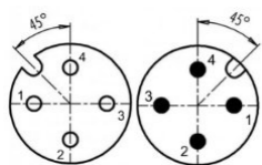
Spiral Verbindungskabel M12A/4p Spiral Connection cable M12A/4p
